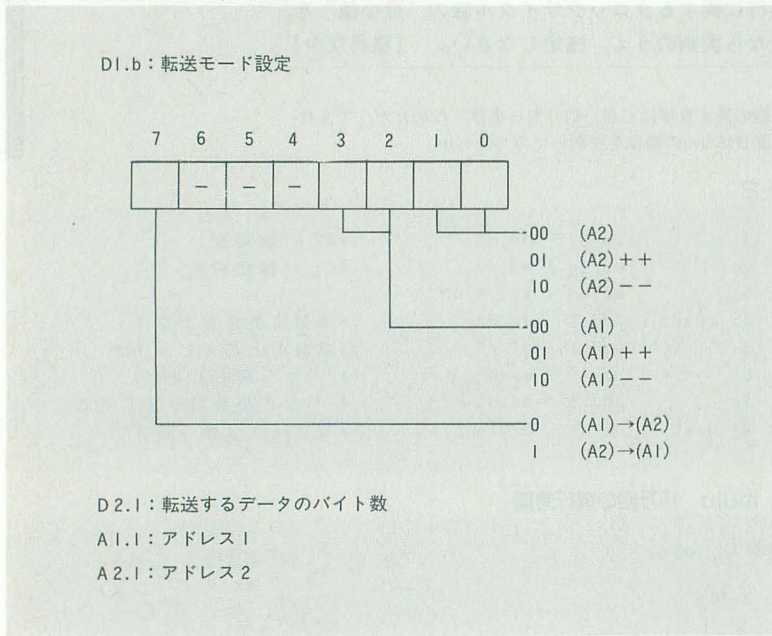
図2 IOCSコール8AHで実行されるプログラム
